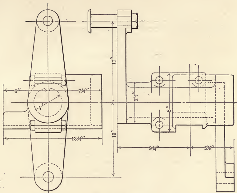
FIG. 45.—Rocker.
