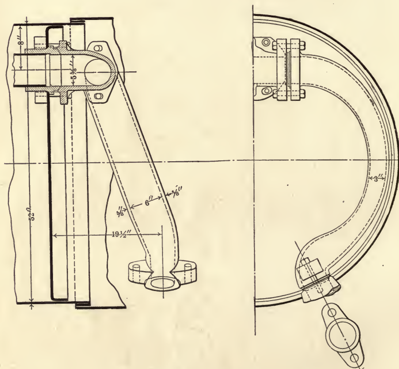
FIG. 33.—Branch-pipe.
