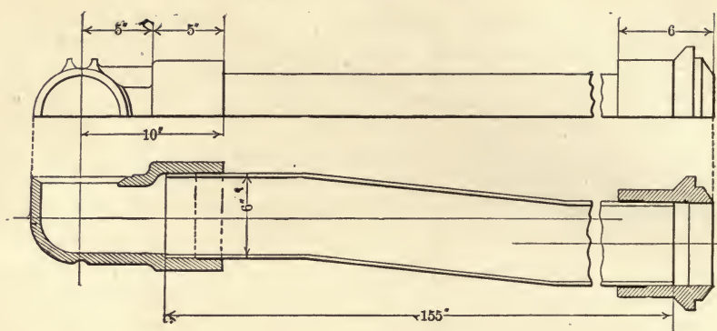
FIG. 32.—Dry-pipe.
